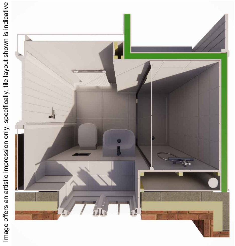
1 Ensuite Layout 1 : 20
