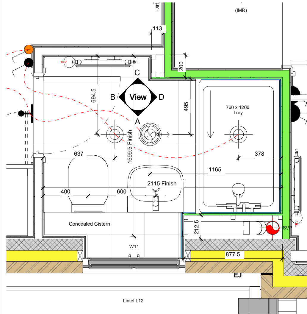
1 Ensuite Layout 1 : 20
